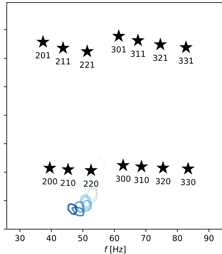
QNM model: 220
