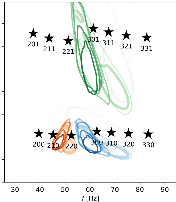
QNM model: 220+221+210
