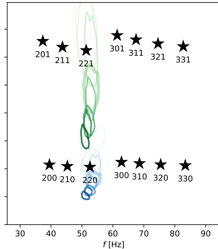
QNM model: 220+221
