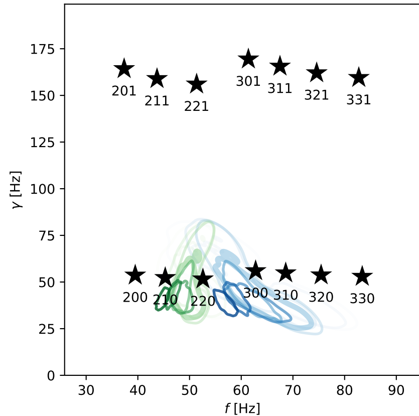
QNM model: 220+210
