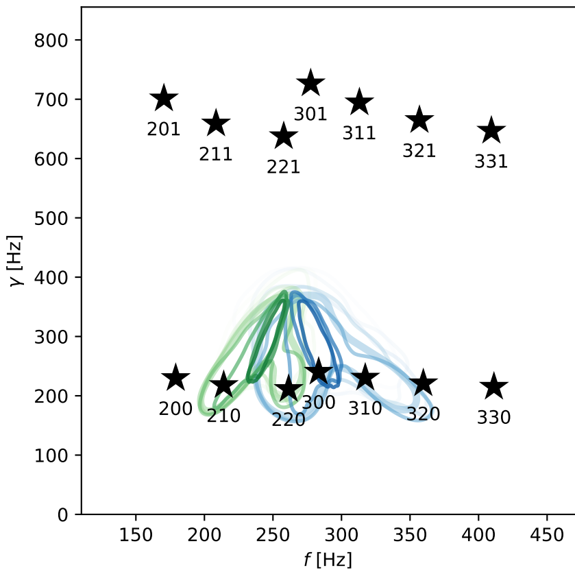
QNM model: 220+210
