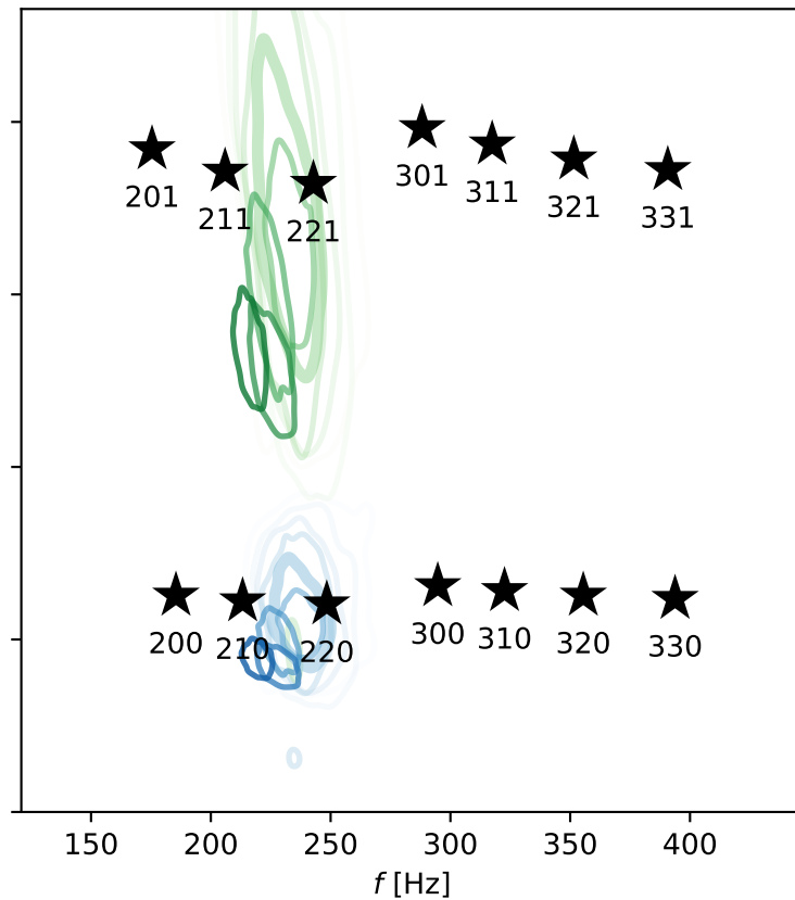
QNM model: 220+221
