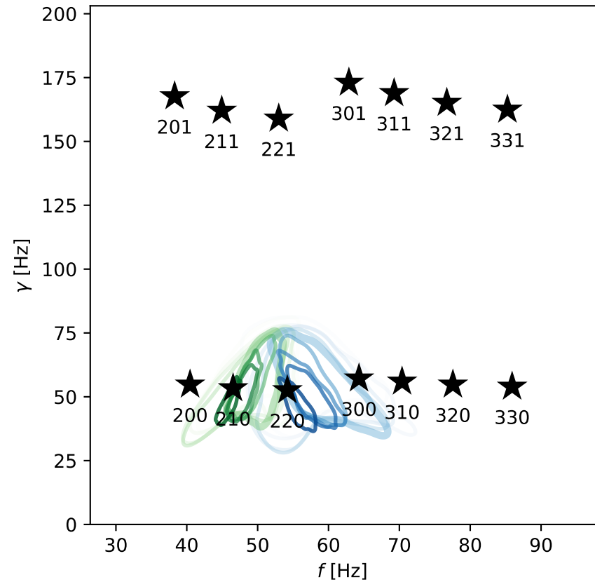
QNM model: 220+210
