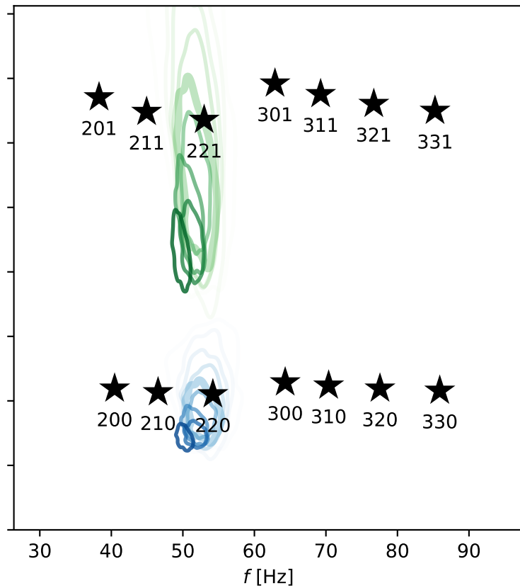
QNM model: 220+221
