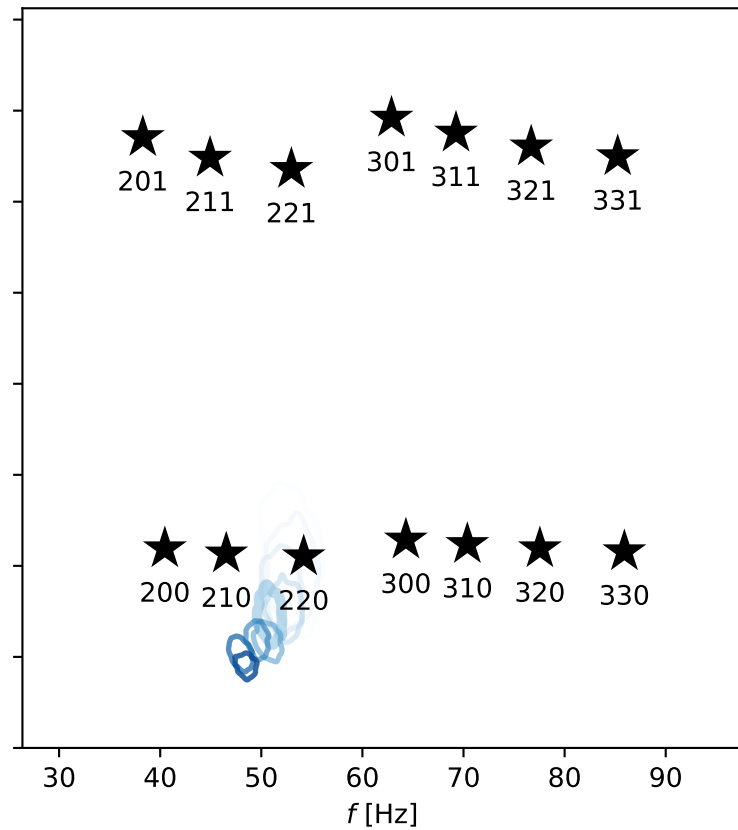
QNM model: 220
