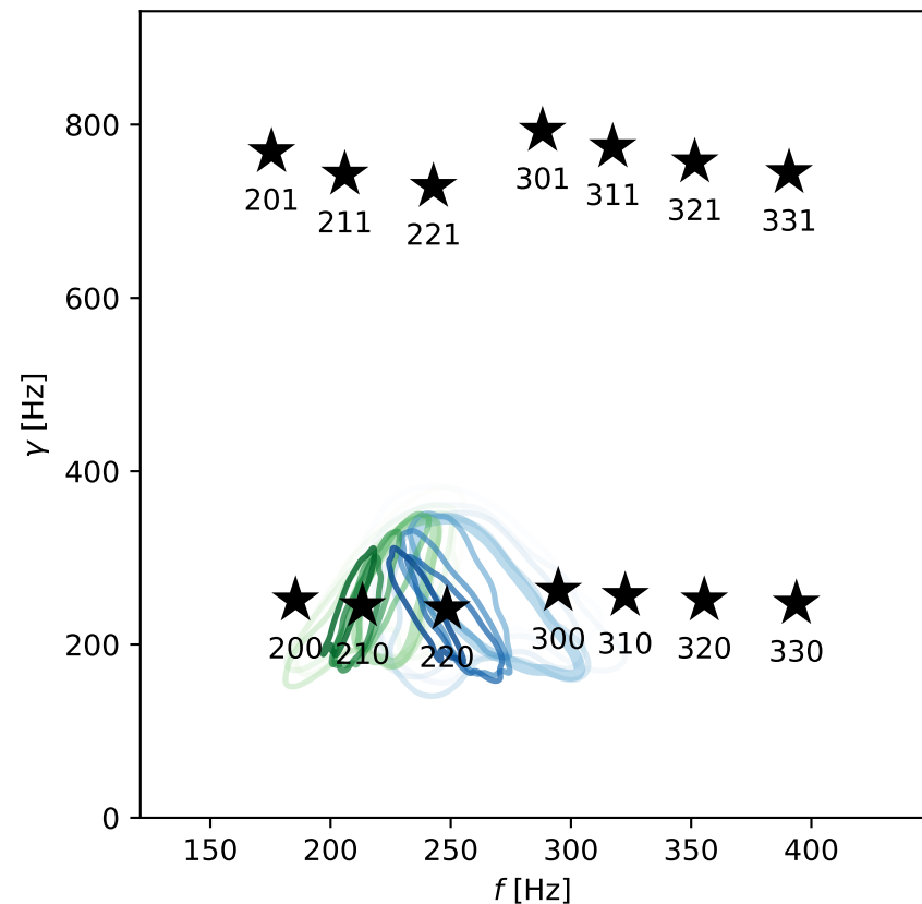
QNM model: 220+210
