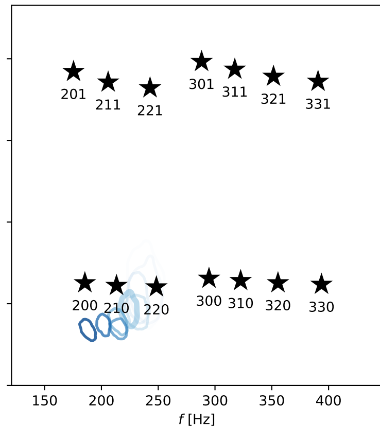
QNM model: 220
