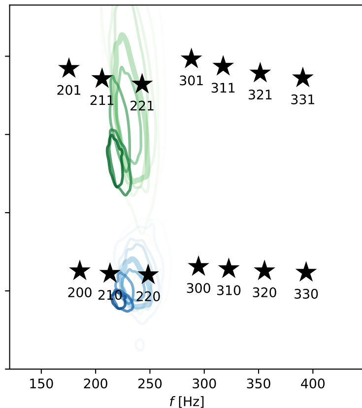
QNM model: 220+221
