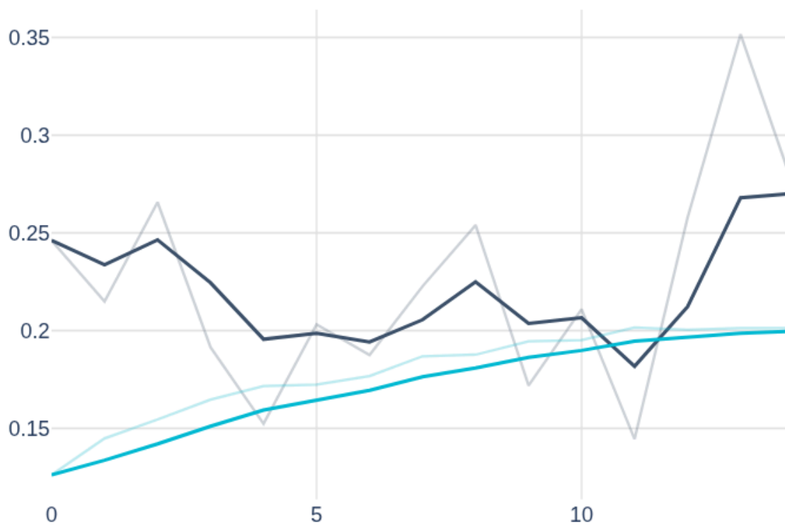
epoch_precision_1
