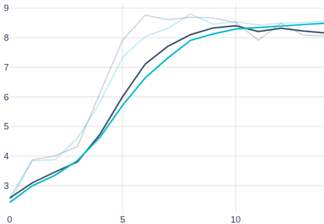
epoch_logit_max
