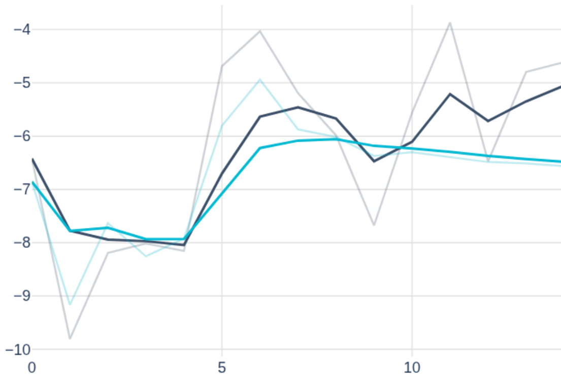
epoch_logit_min
