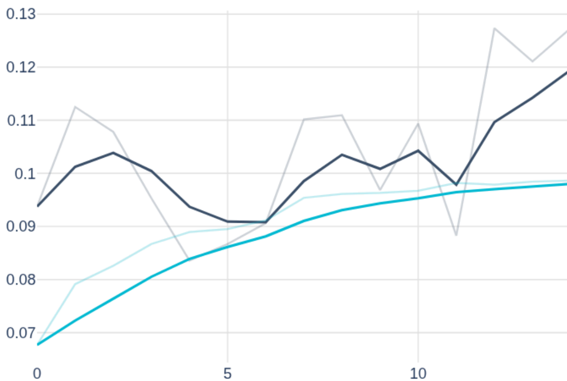
epoch_precision_5
