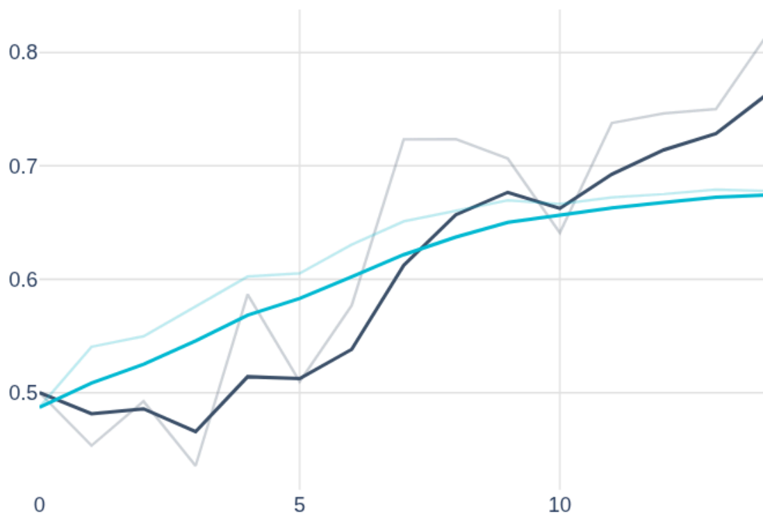
epoch_recall_torso_20
