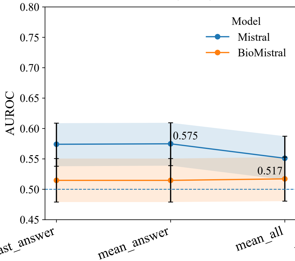
MedQA (MCQ)
