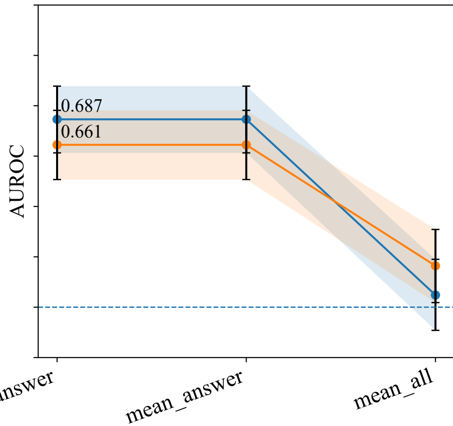
PubMedQA (Yes/No/Maybe)
