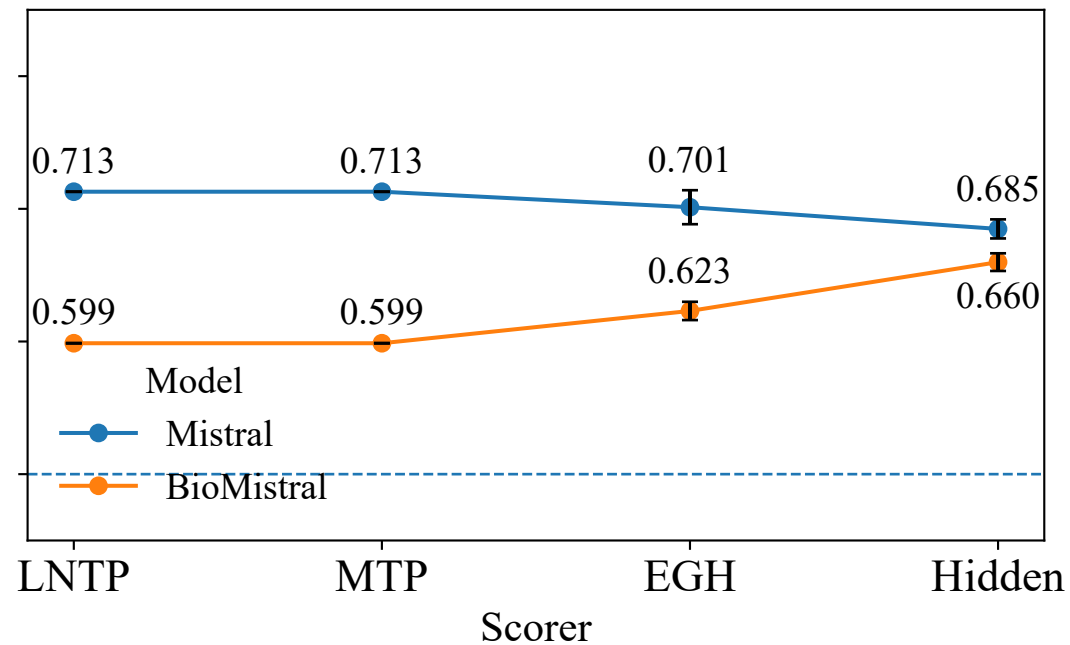
PubMedQA (Yes/No/Maybe)
