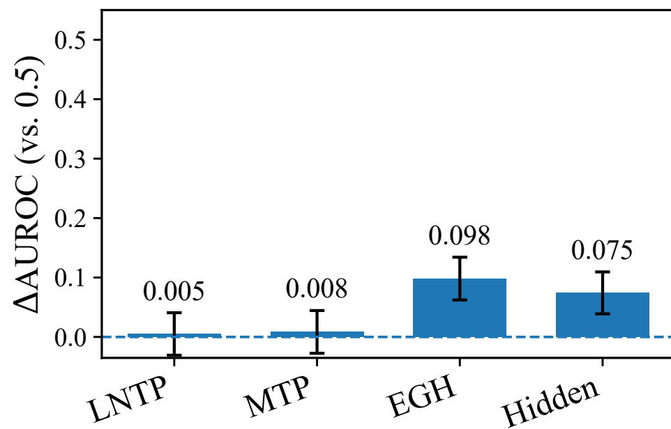
MedQA (MCQ)
