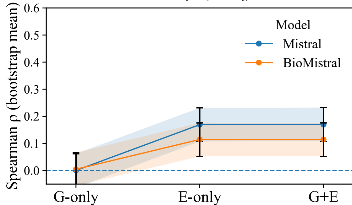
MedQA (MCQ)
