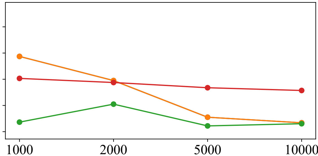
PubMedQA (Yes/No/Maybe)
