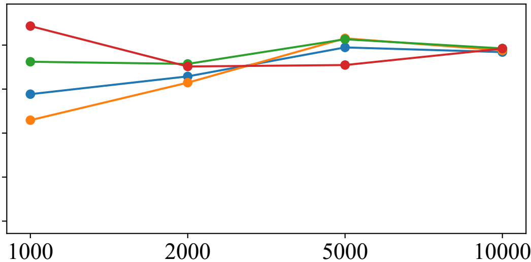
MedQA (MCQ)
