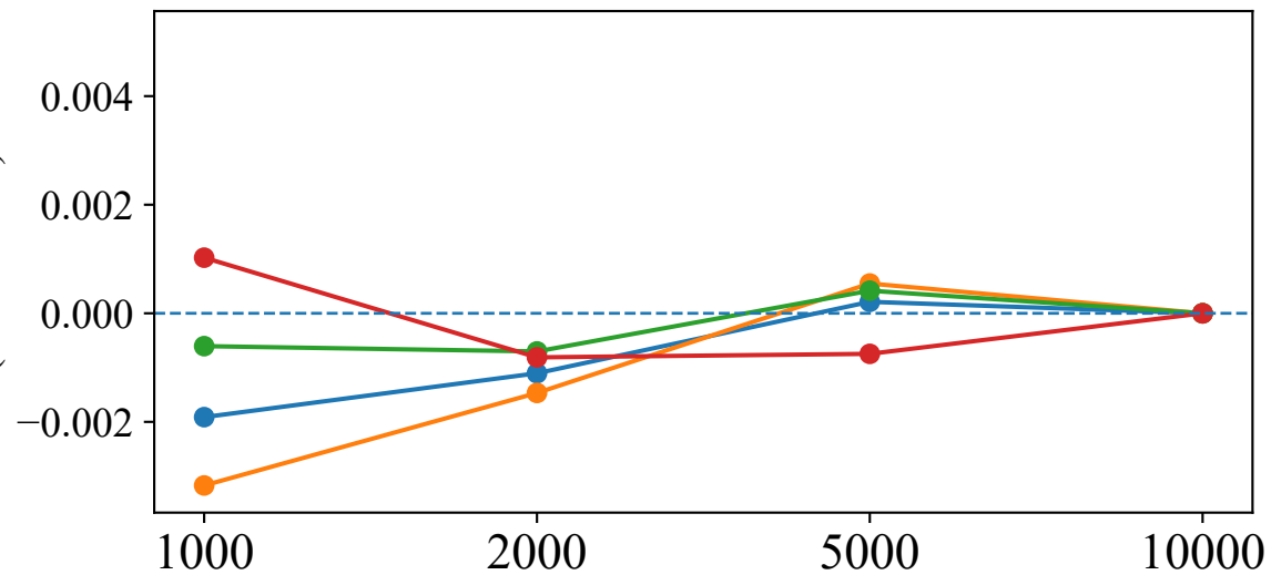
MedQA (MCQ)
