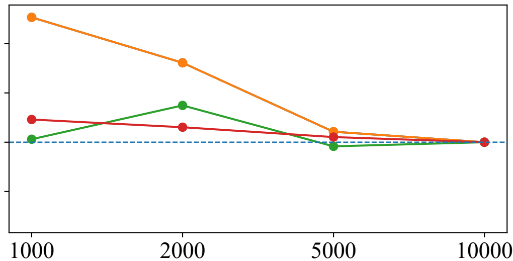
PubMedQA (Yes/No/Maybe)
