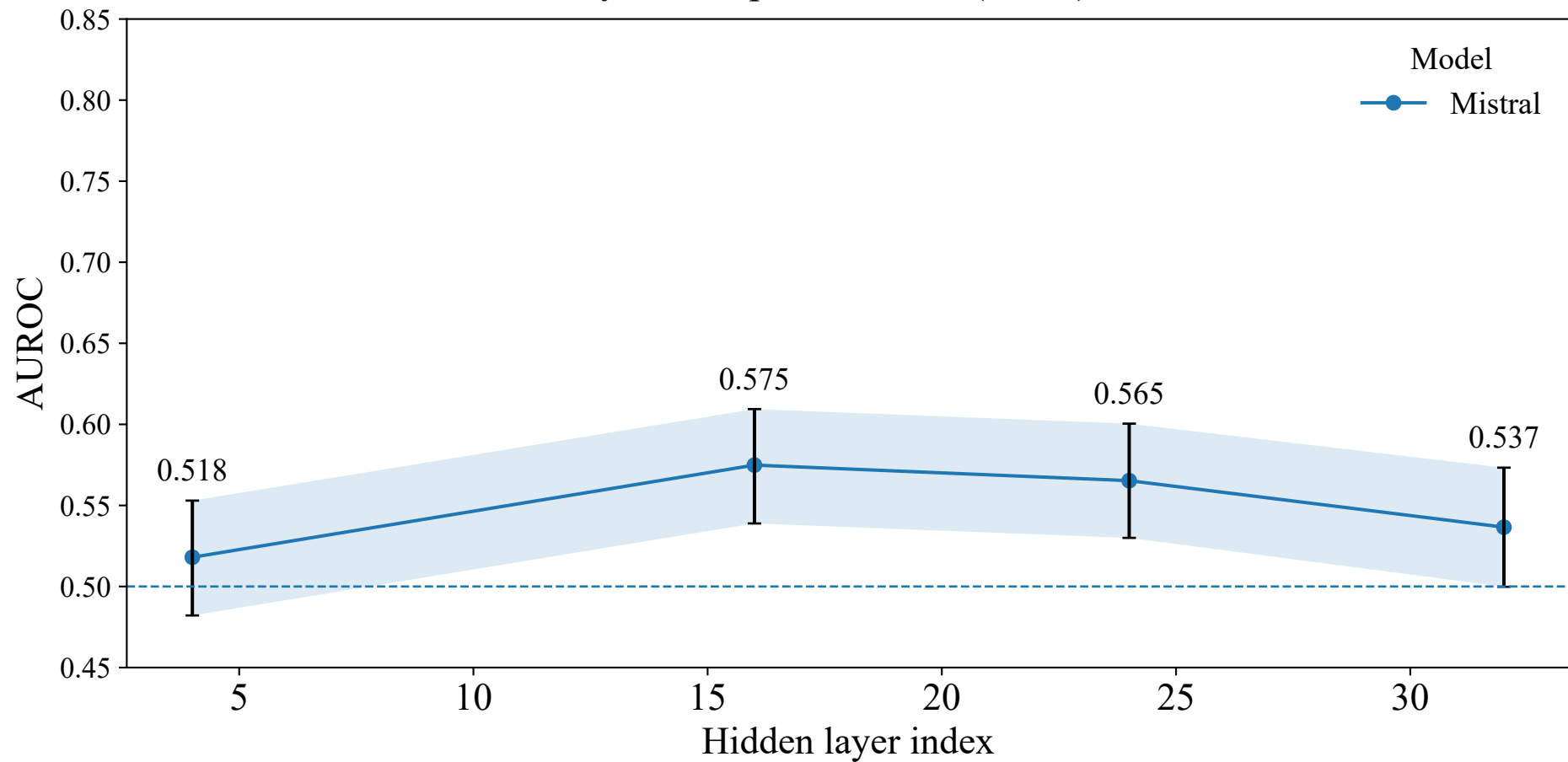
Hidden Layer Sweep — MedQA (MCQ) — Mistral
