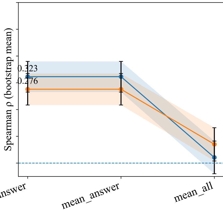
PubMedQA (Yes/No/Maybe)
