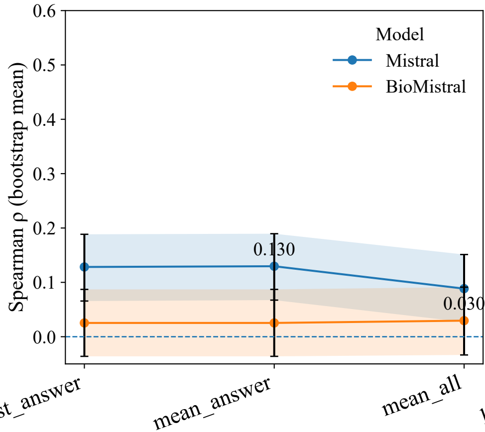
MedQA (MCQ)
