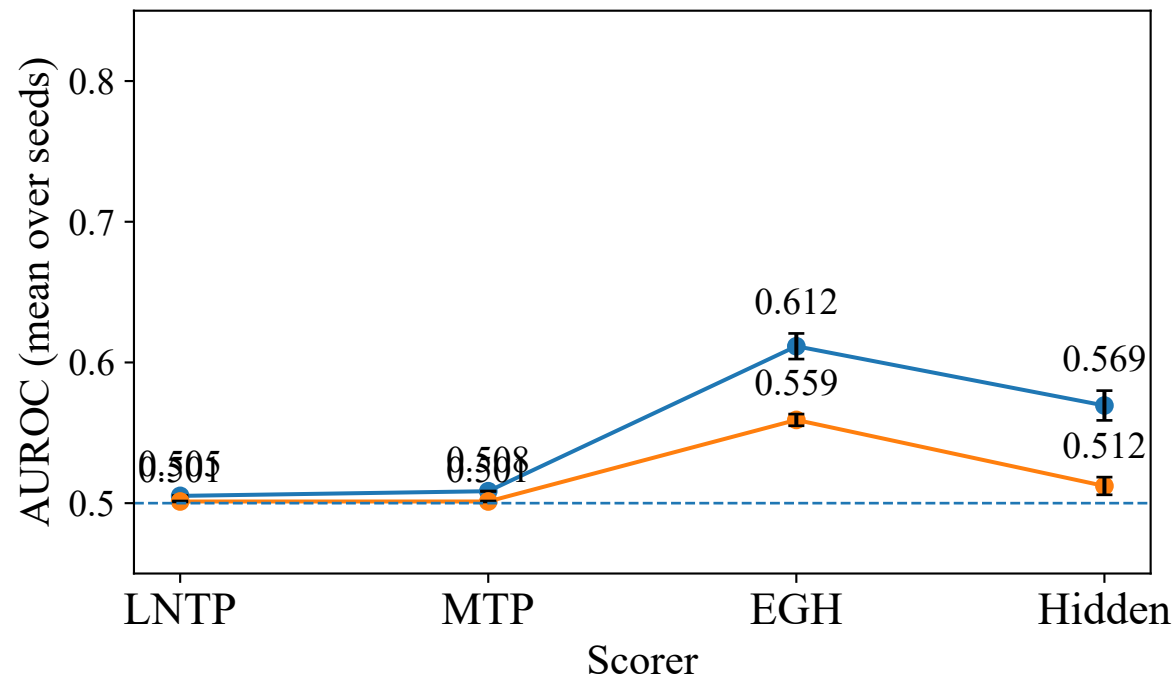
MedQA (MCQ)
