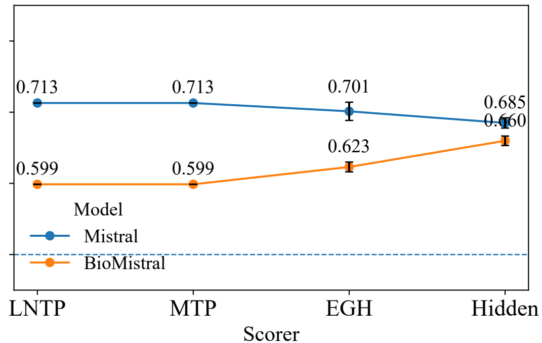
PubMedQA (Yes/No/Maybe)
