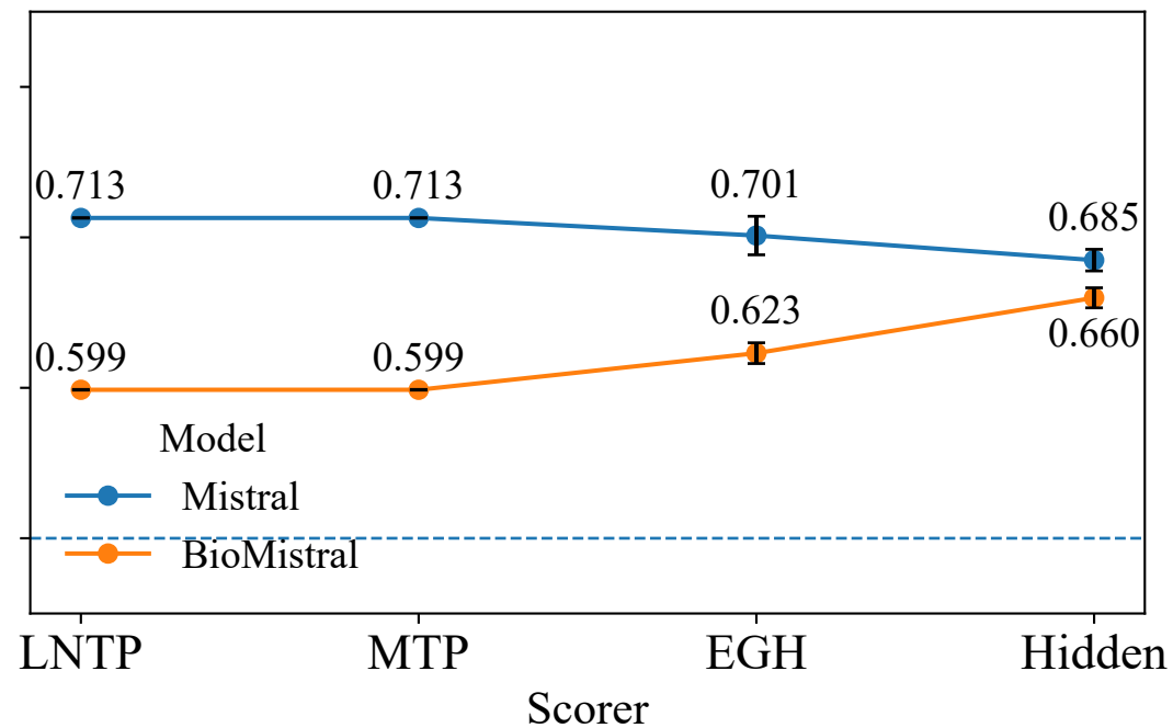
PubMedQA (Yes/No/Maybe)
