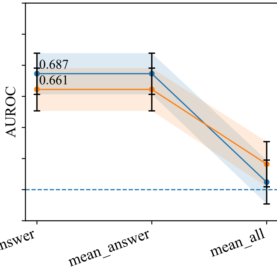
PubMedQA (Yes/No/Maybe)
