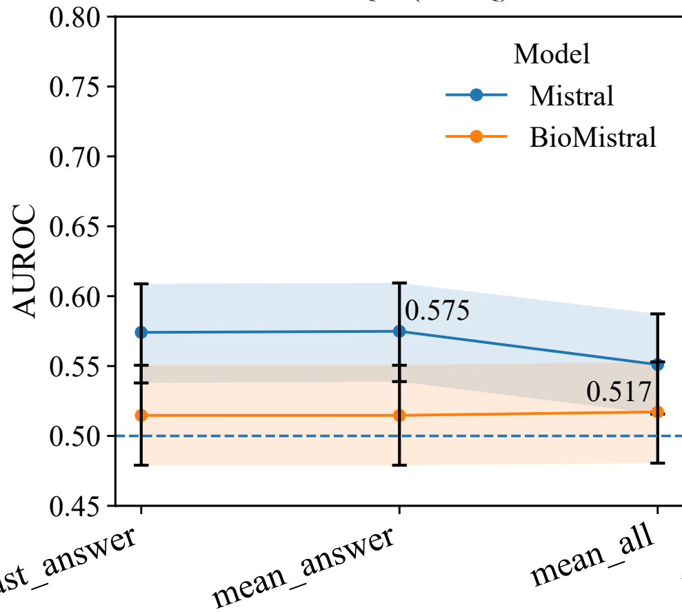
MedQA (MCQ)
