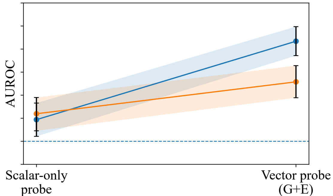
PubMedQA (Yes/No/Maybe)
