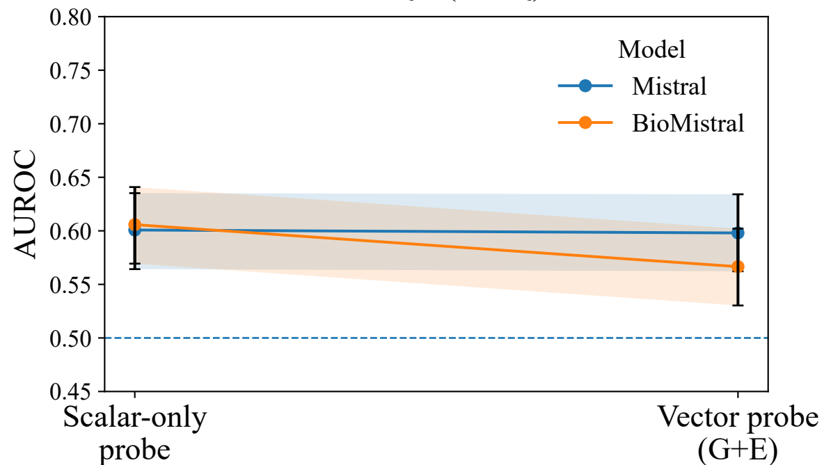
MedQA (MCQ)
