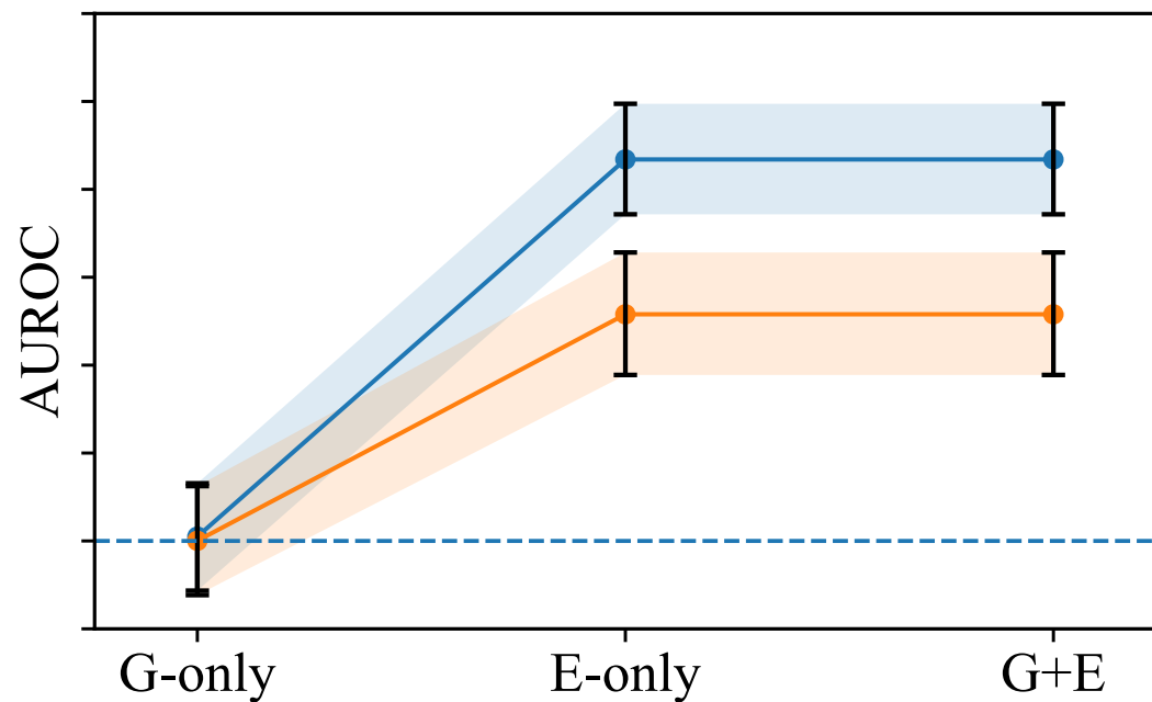
PubMedQA (Yes/No/Maybe)
