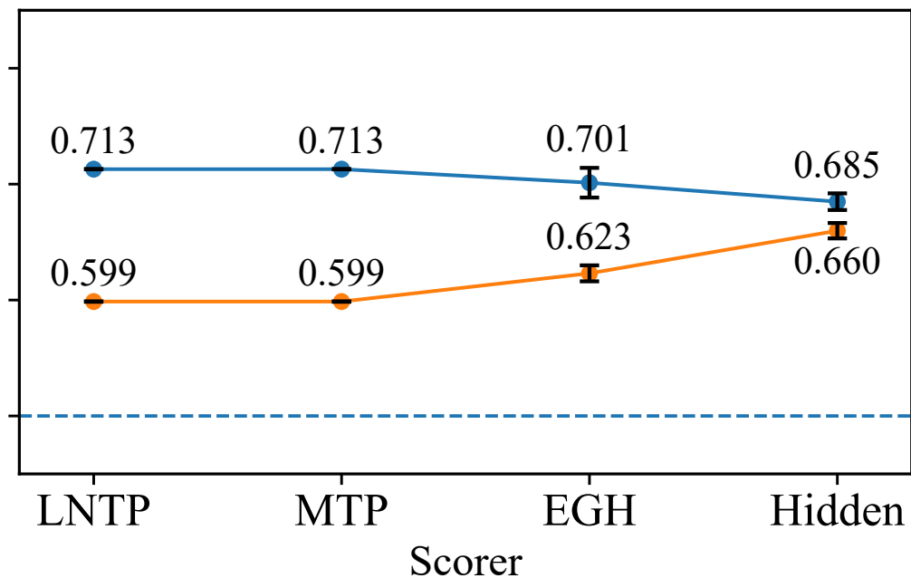
PubMedQA (Yes/No/Maybe)
