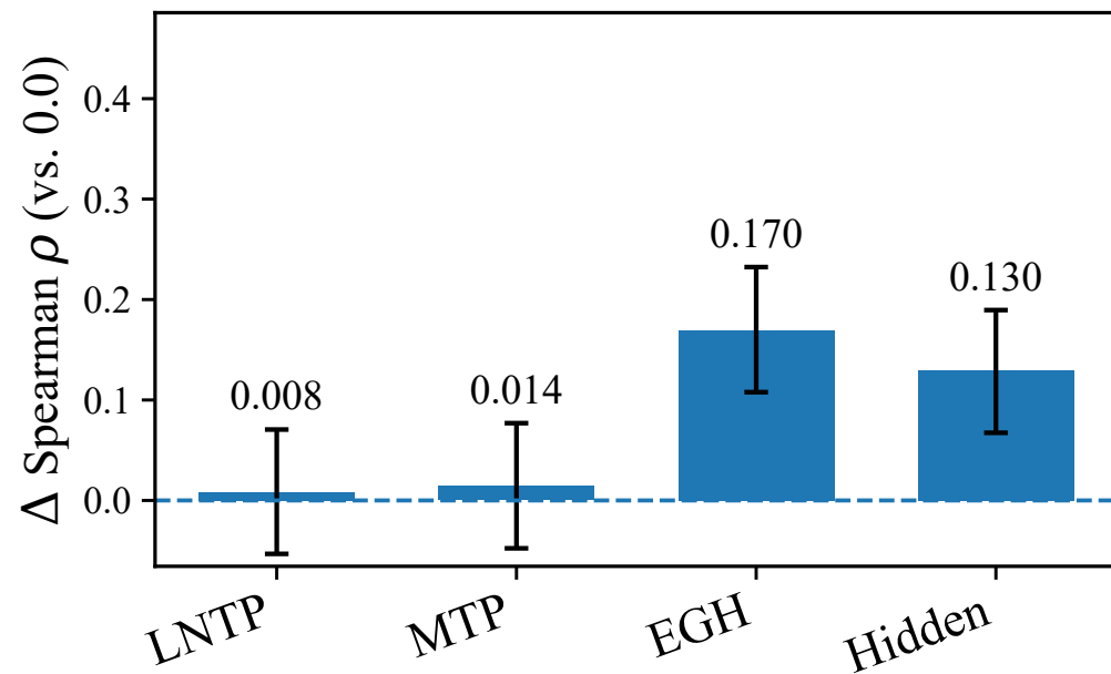
MedQA (MCQ)
