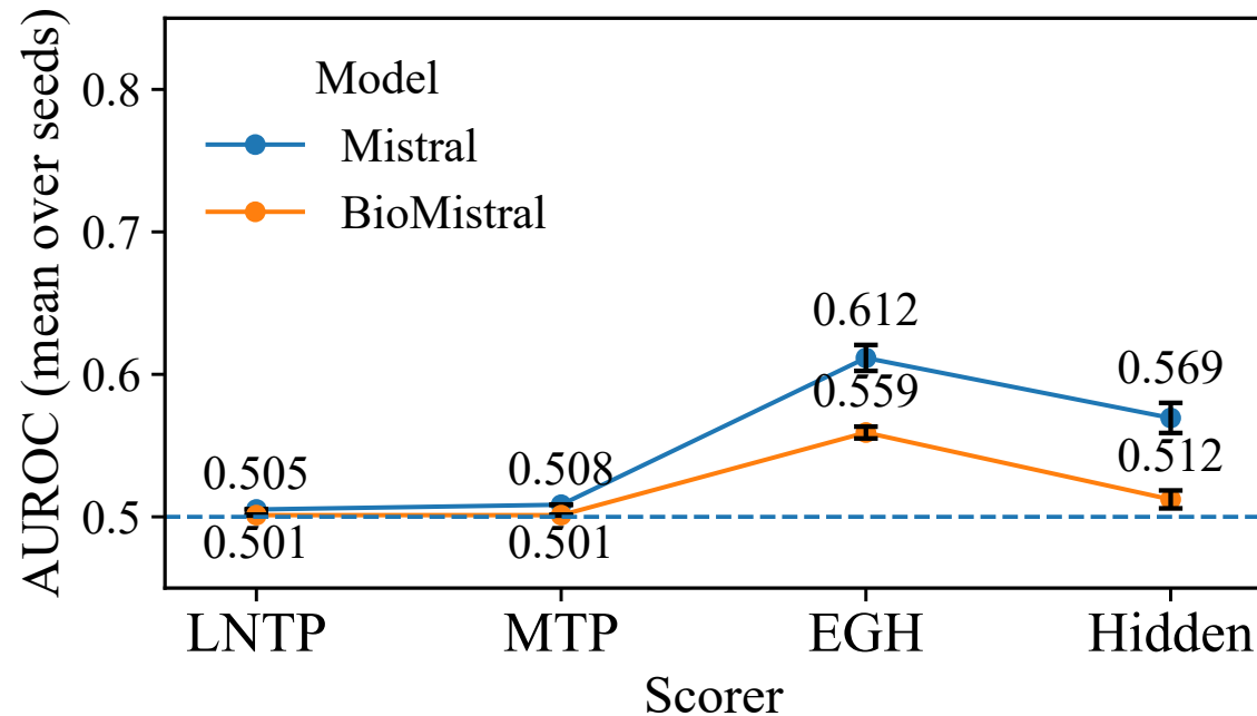
MedQA (MCQ)
