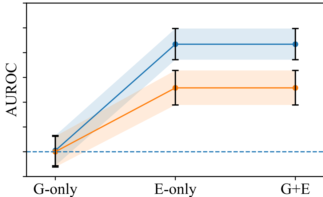
PubMedQA (Yes/No/Maybe)
