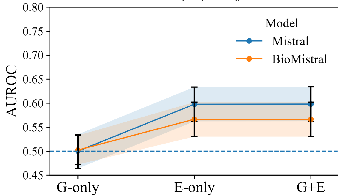
MedQA (MCQ)
