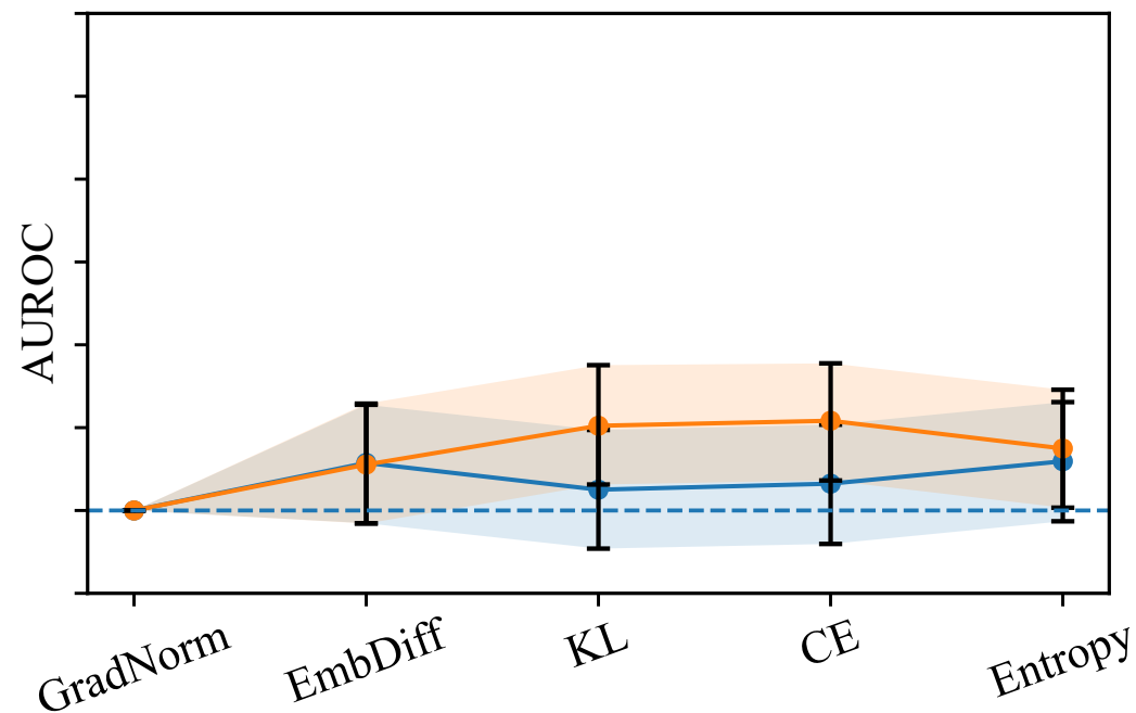
PubMedQA (Yes/No/Maybe)
