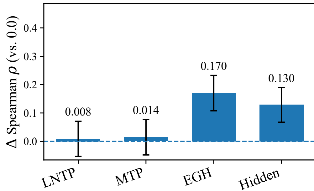
MedQA (MCQ)
