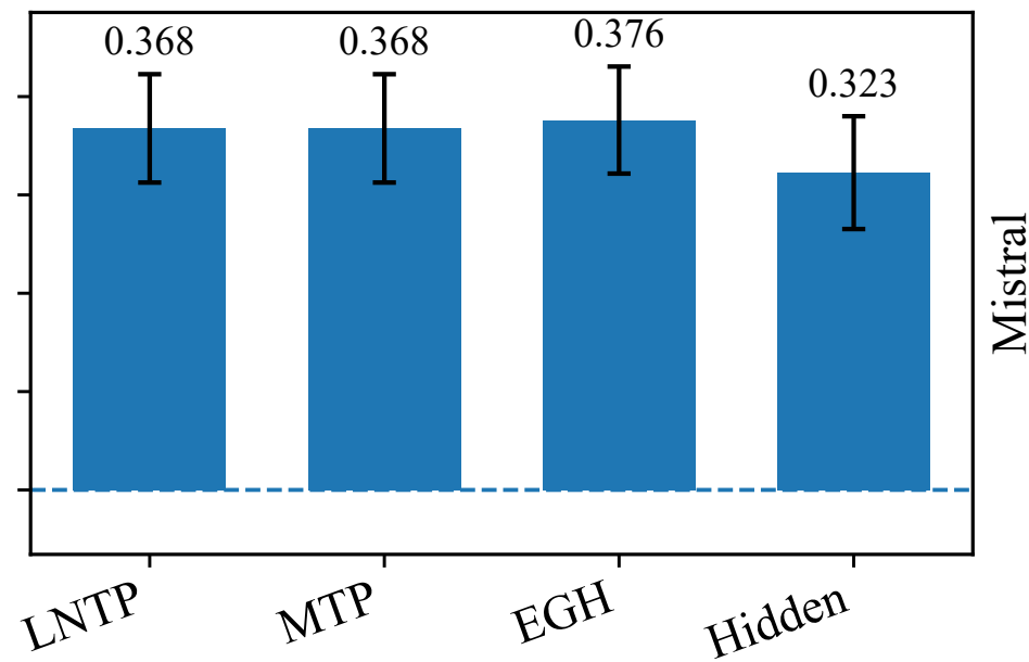
PubMedQA (Yes/No/Maybe)
