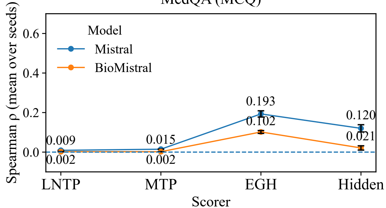
MedQA (MCQ)
