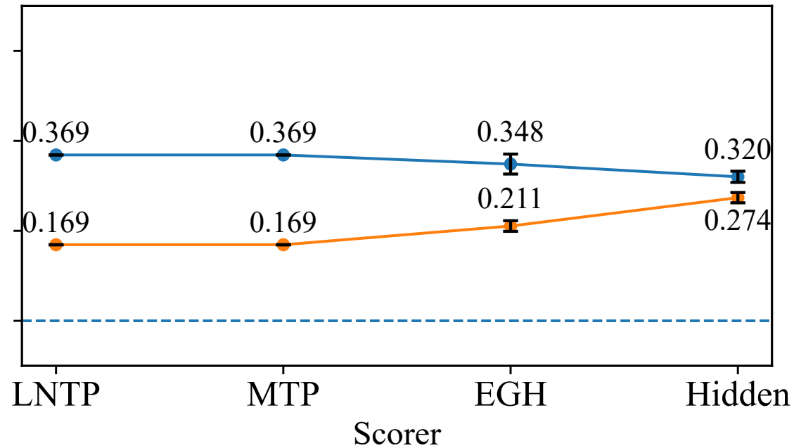
PubMedQA (Yes/No/Maybe)
