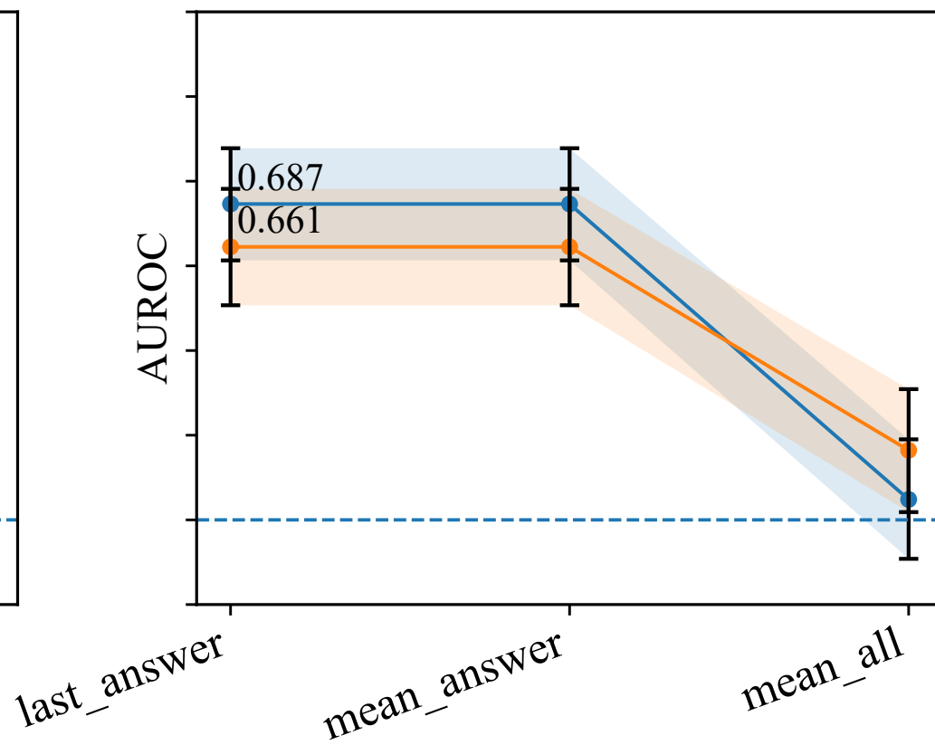
PubMedQA (Yes/No/Maybe)
