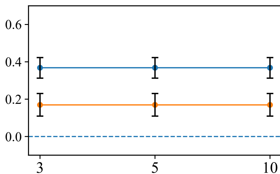
PubMedQA (Yes/No/Maybe)
