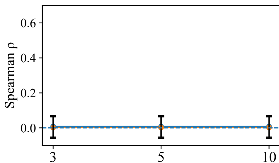
MedQA (MCQ)
