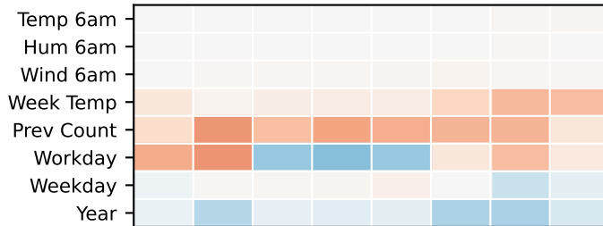
SHAP
