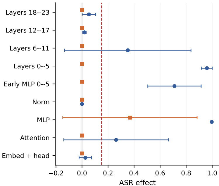
Pythia 410M
