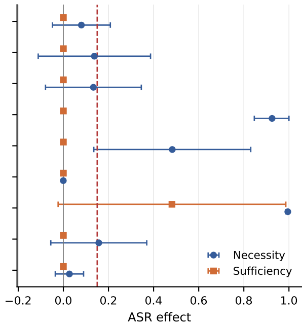
Pythia 1.4B
