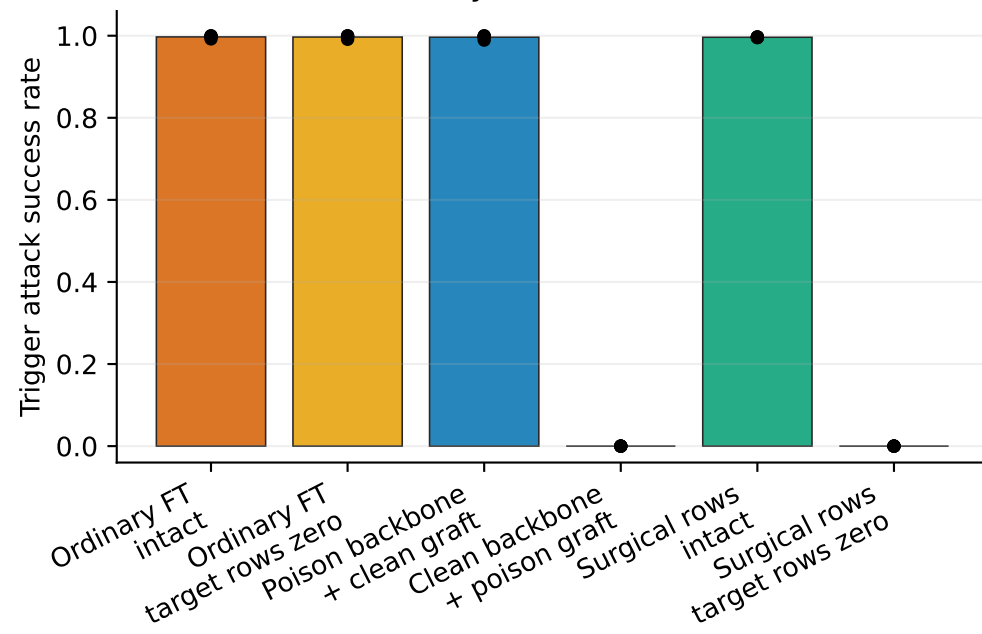
Pythia-410m
