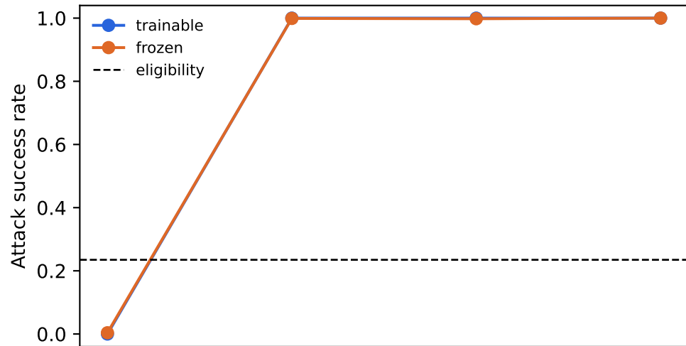
pythia-410m
