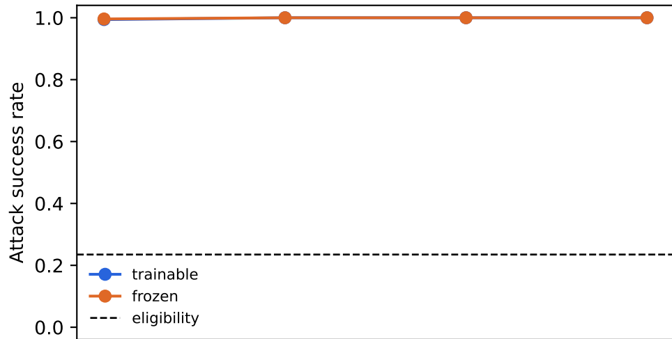
pythia-1.4b
