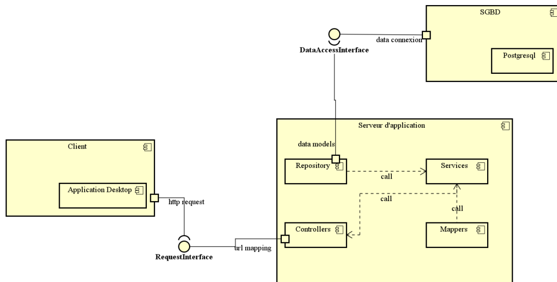
Figure 35 diagramme de composant du système.
