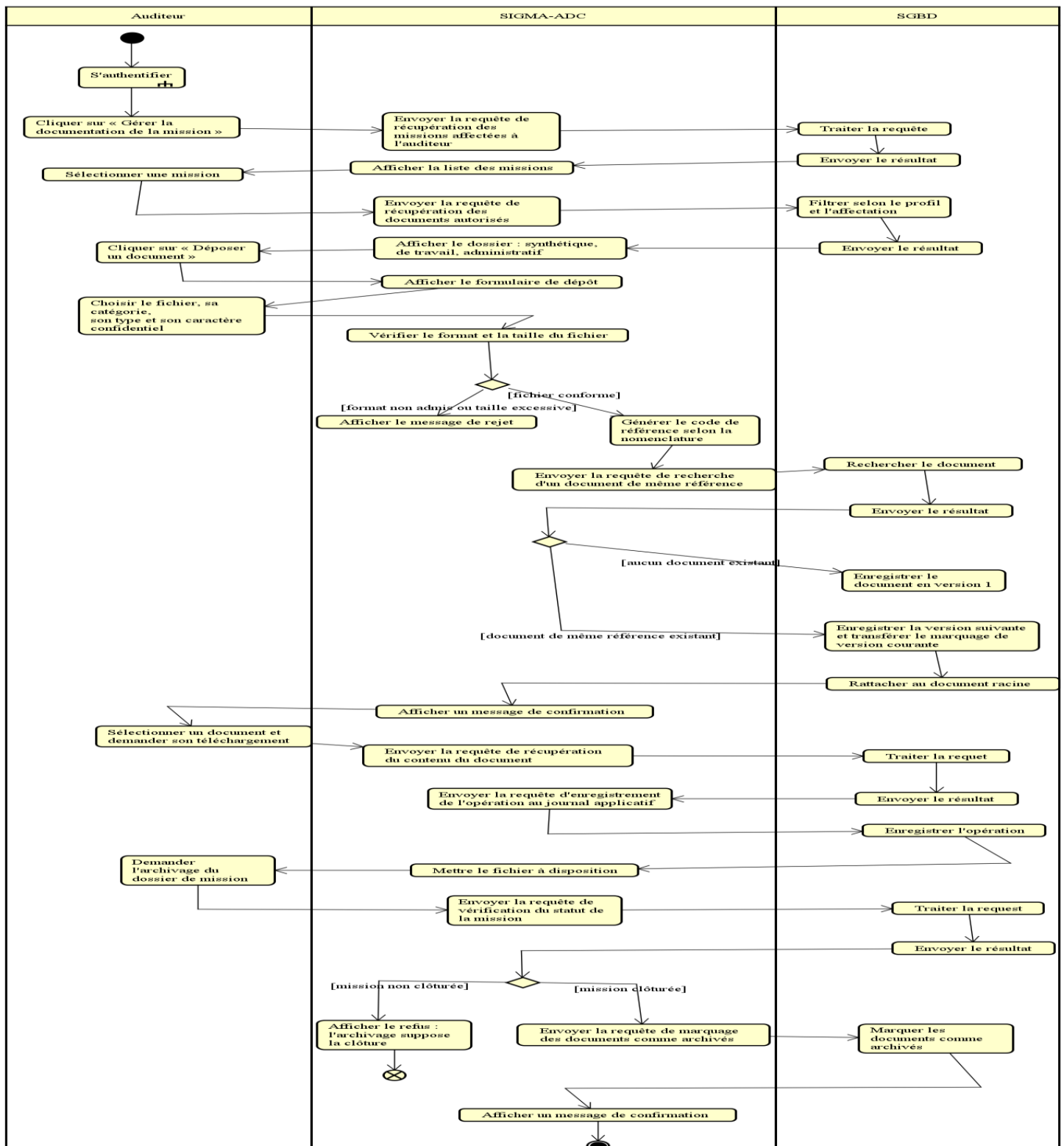
Figure 24 diagramme d'activité du cas : Gérer la documentation de la mission
