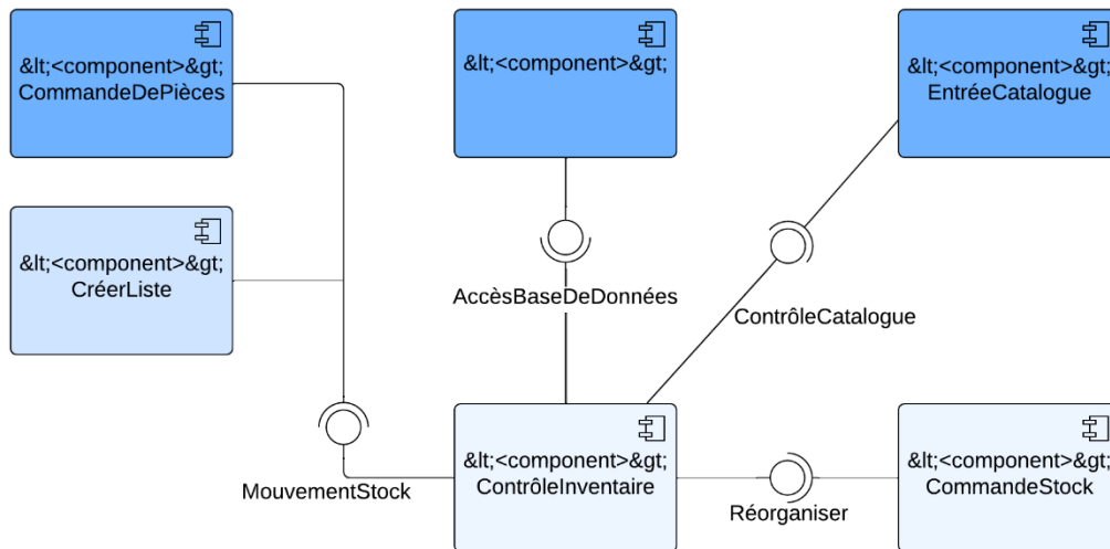
Figure 34 exemple de diagramme de composant
