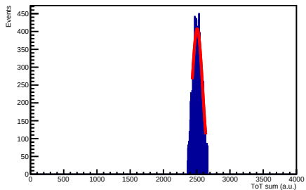
Run 179 ToT sum
