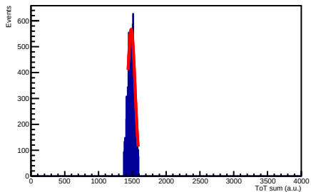
Run 176 ToT sum
