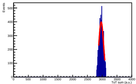
Run 180 ToT sum
