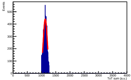
Run 175 ToT sum
