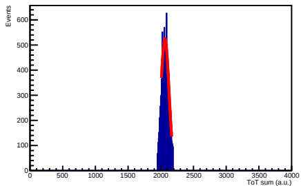
Run 178 ToT sum
