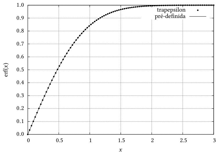
Figura 4.6: Função \text{erf}(x) calculada por integração numérica, com \text{trapepsilon} e \epsilon = 1 \times 10^{-6} , versus a \text{erf} pré-definida no programa de plotagem.
