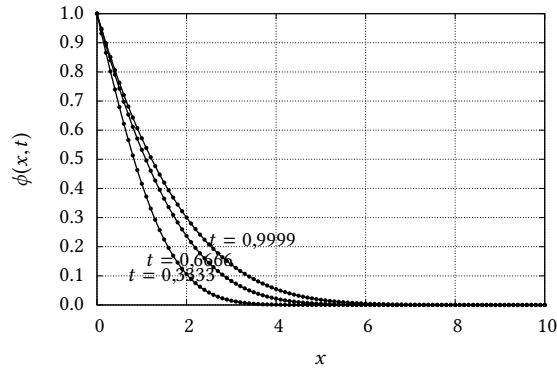
Figura 14.12: Comparação entre as soluções analítica (linhas) e numérica com um esquema implícito (pontos) da equação da difusão-advectação com termo de decaimento, para t = 0,333 , t = 0,666 e t = 0,999 .
