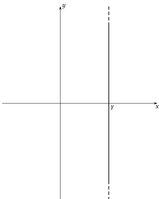
Figura 12.3: Caminho de integração para a fórmula de inversão 12.14 .
