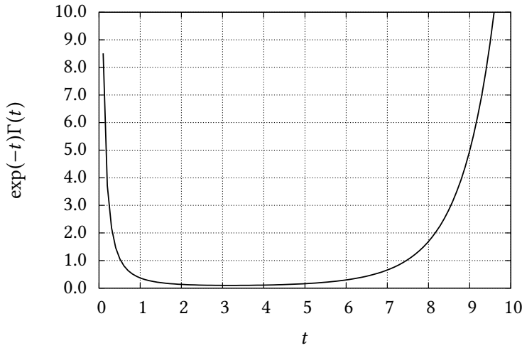
Figura 12.1: Gráfico da função e^{-t}\Gamma(t) .
