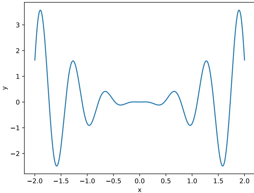
non convex function
