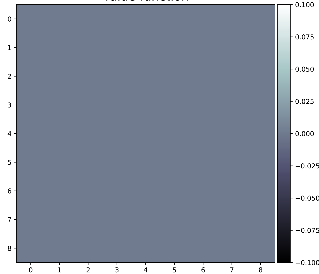
Value function
