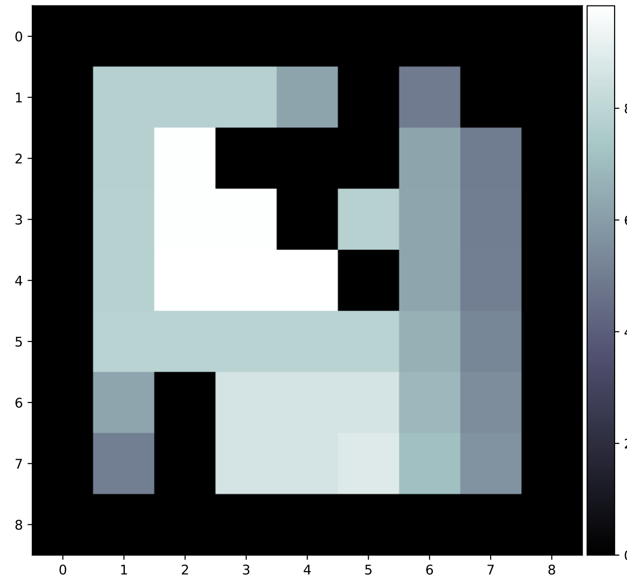
Value function
