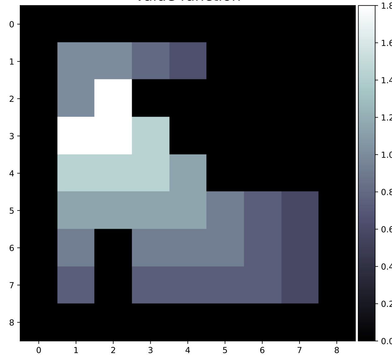
Value function
