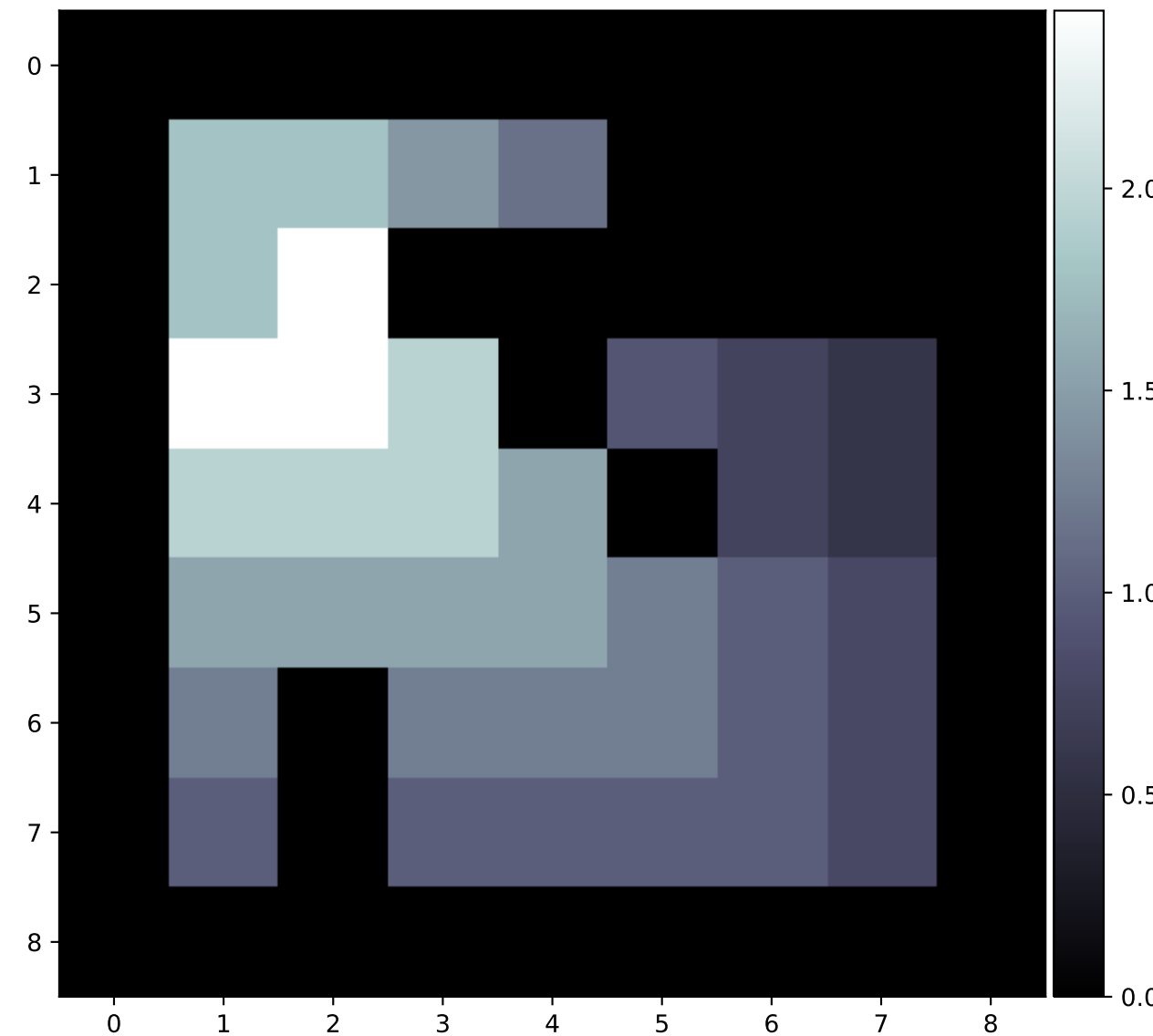
Value function
