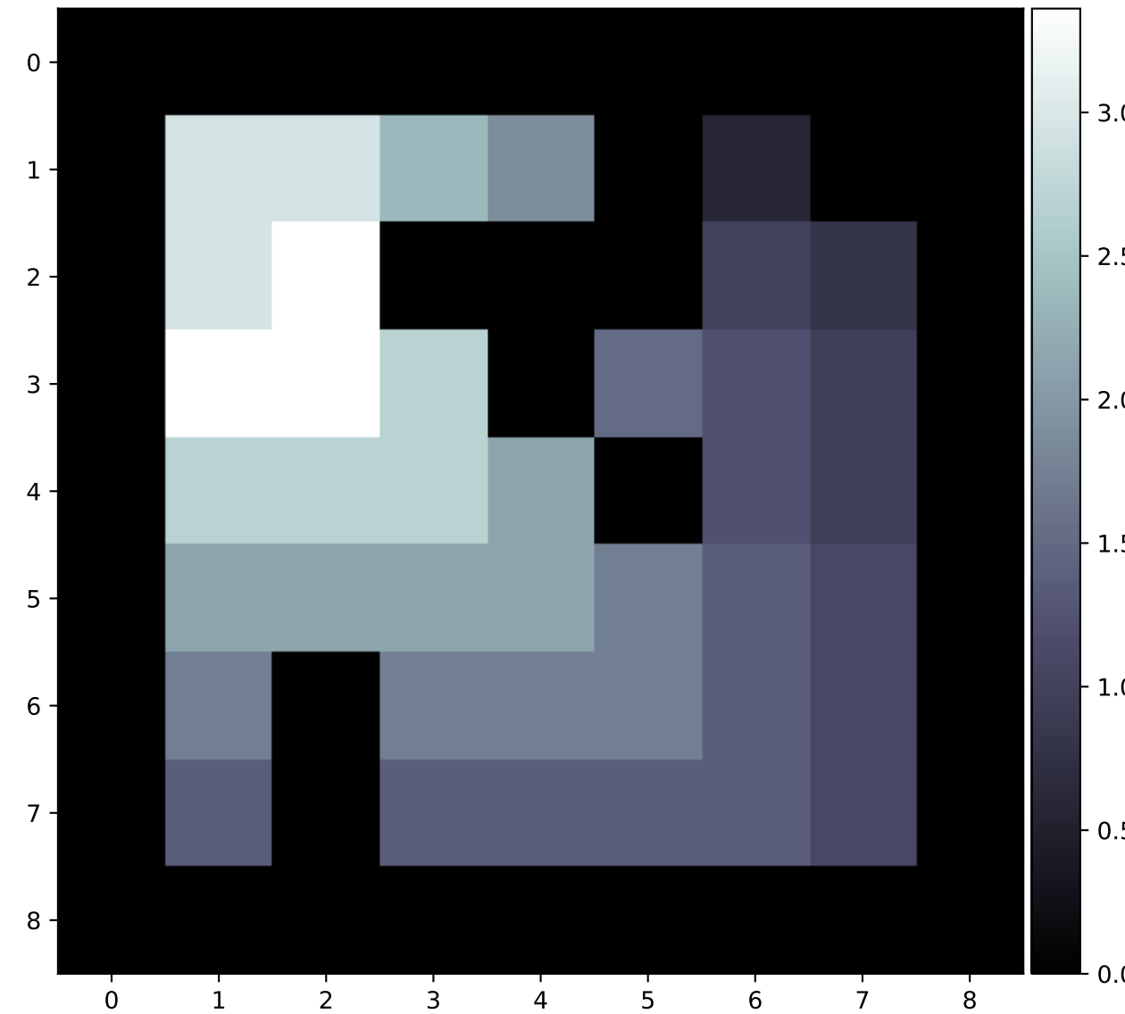
Value function
