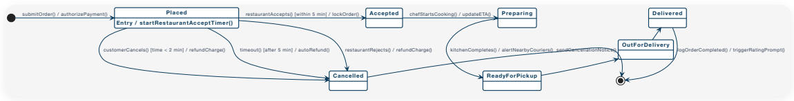
圖 3.2 QuickBite 訂單生命週期狀態機圖 (State Machine Diagram)
