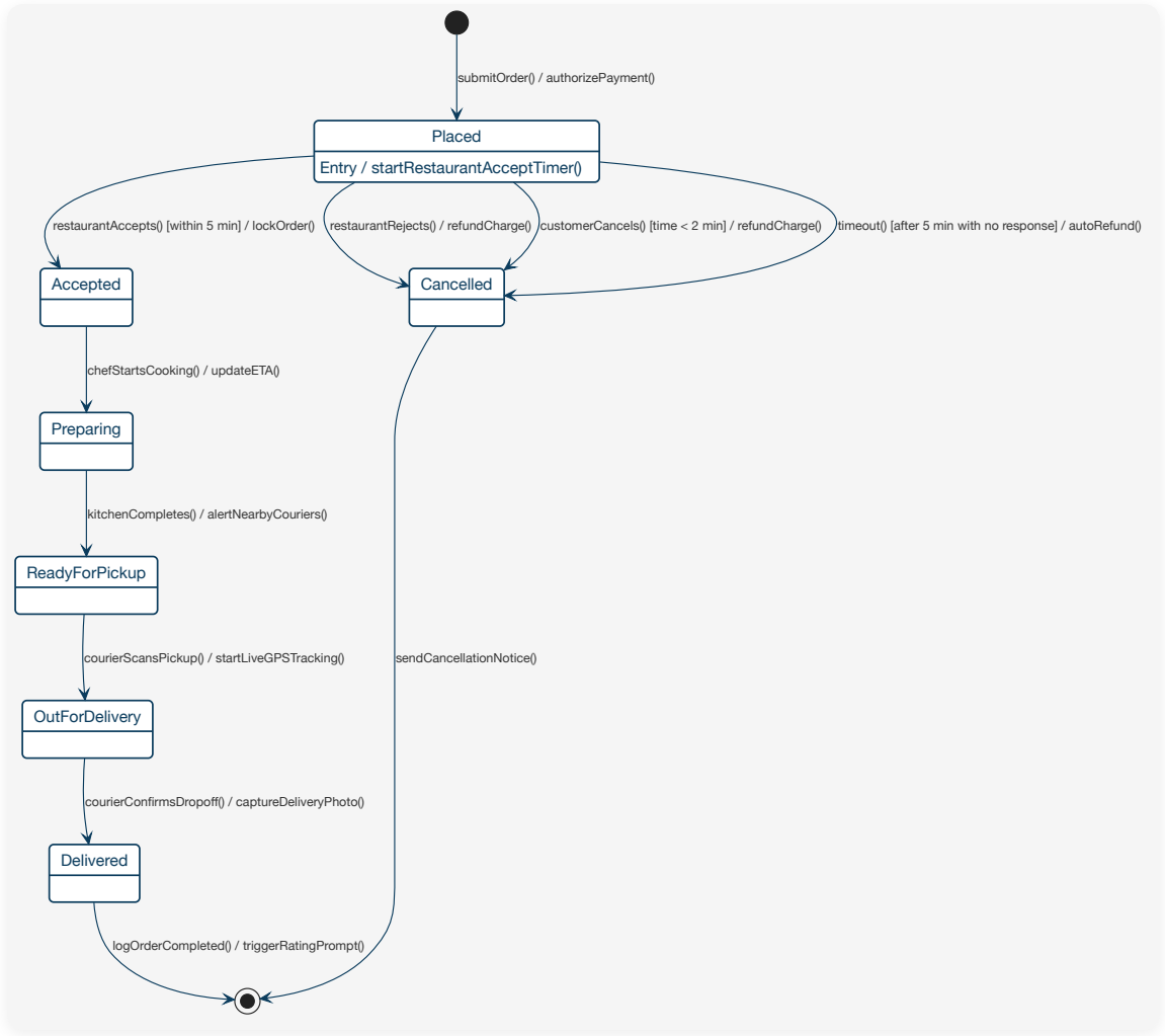
圖 3.2 QuickBite 訂單生命週期狀態機圖 (State Machine Diagram)
