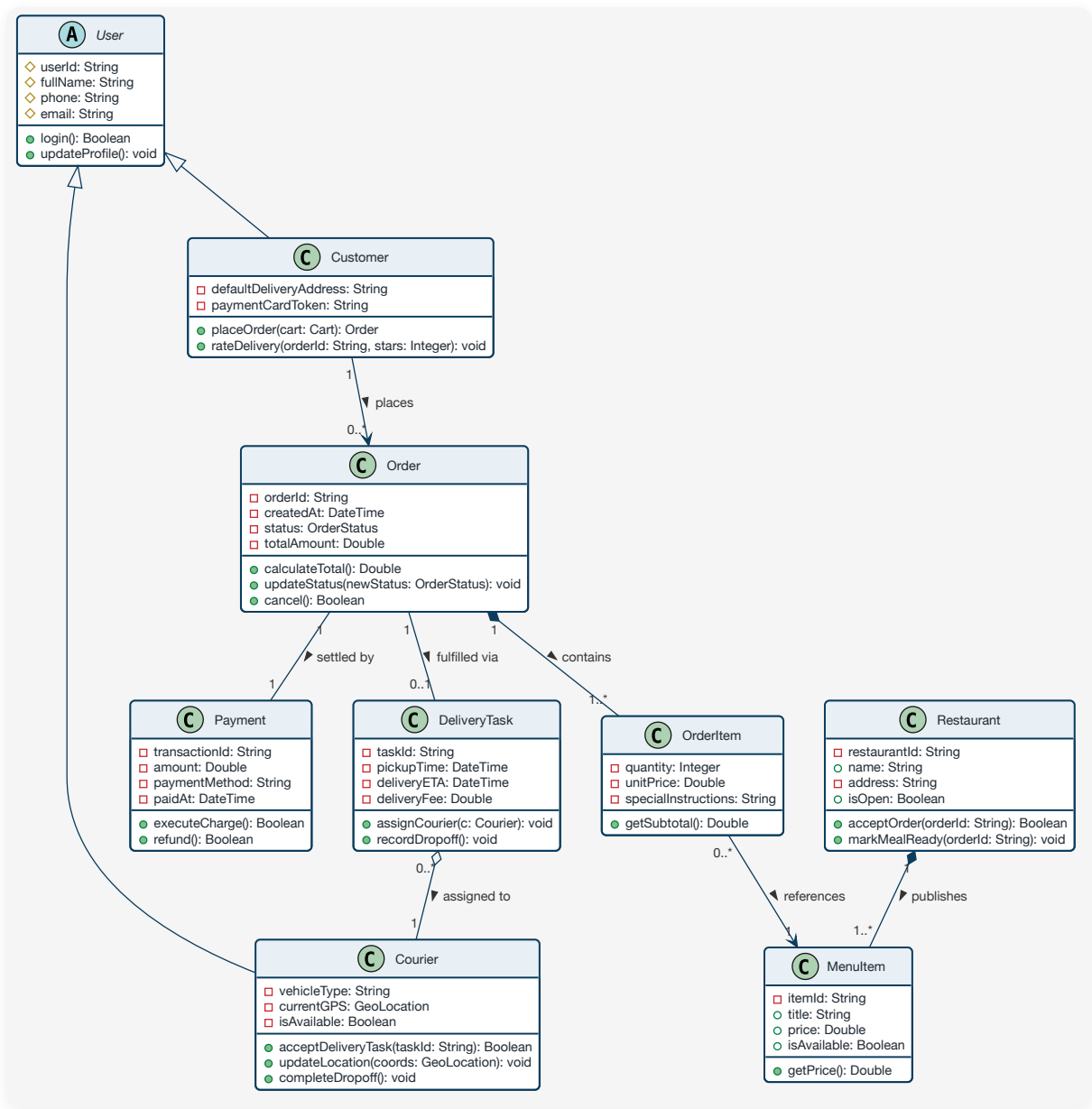
圖 2.1 QuickBite 美食外送平台 UML 領域類別圖 (Class Diagram)
