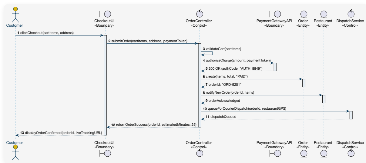
圖 3.1 QuickBite 端到端下單、金流與智慧派單循序圖 (Sequence Diagram)
