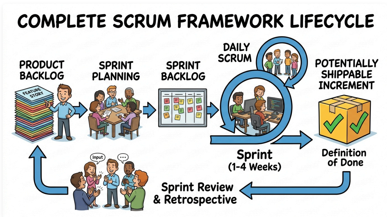
圖 2.5.2：Scrum 完整生命週期。PO 梳理產品待辦清單，團隊在衝刺規劃中拉取任務，於 1~4 週封閉衝刺中透過每日立會對齊進度，最終交付通過 DoD 的增量，經由審查會議演示並在回顧會議中自我改進。
