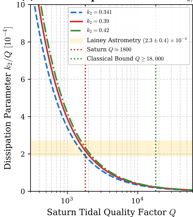
(a) Tidal Dissipation Parameter k_2/Q
