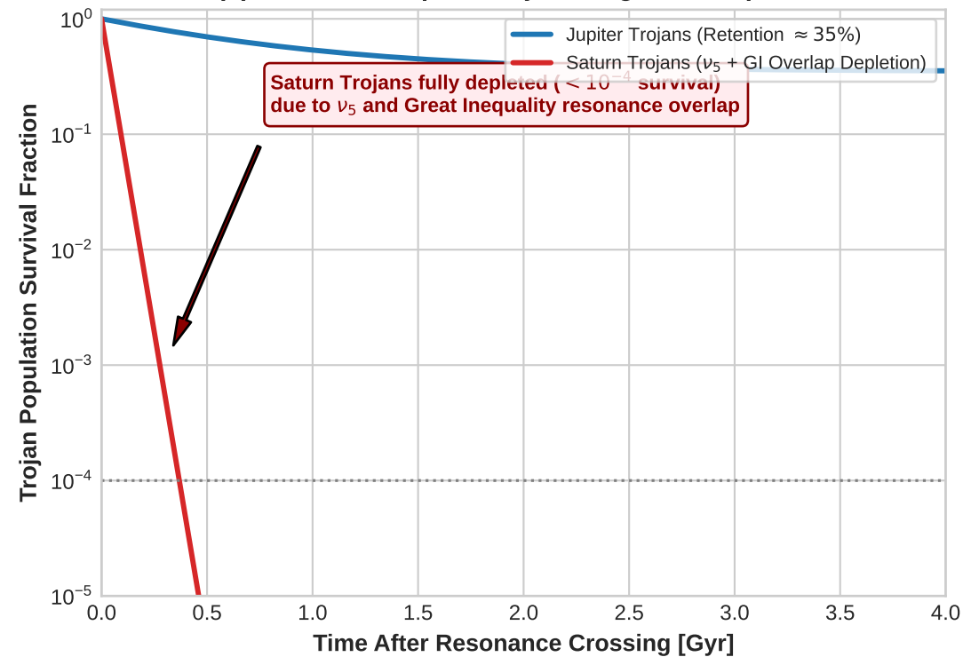
(d) Saturn vs. Jupiter Trojan Long-Term Depletion
