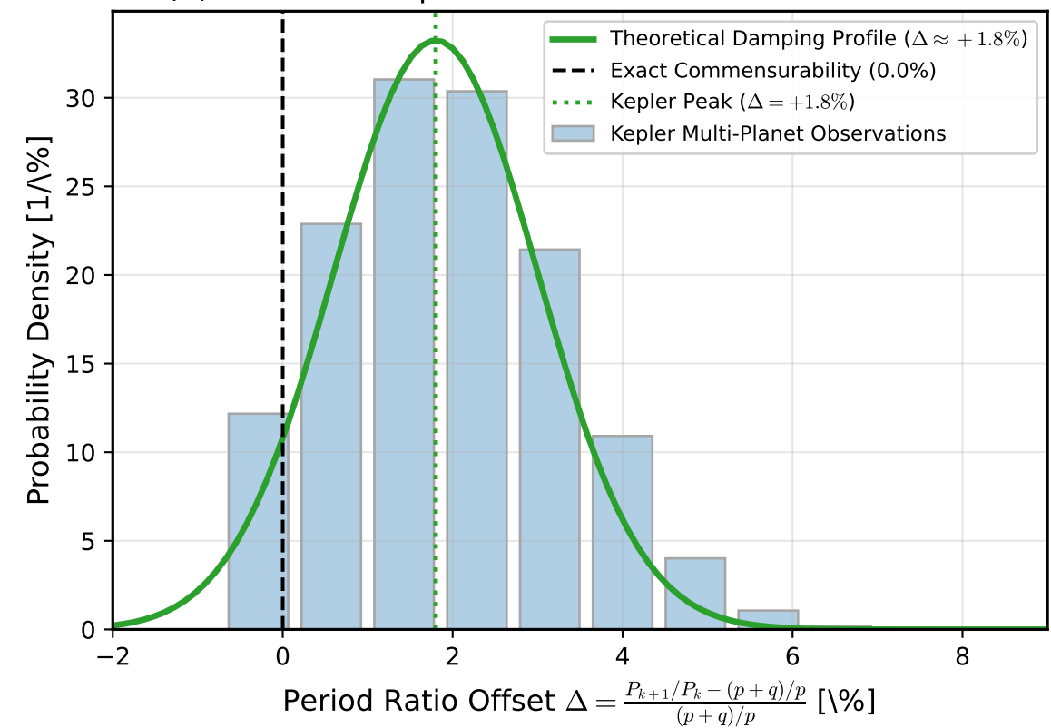
(d) Post-Gas Dispersal Resonance Offset Distribution
