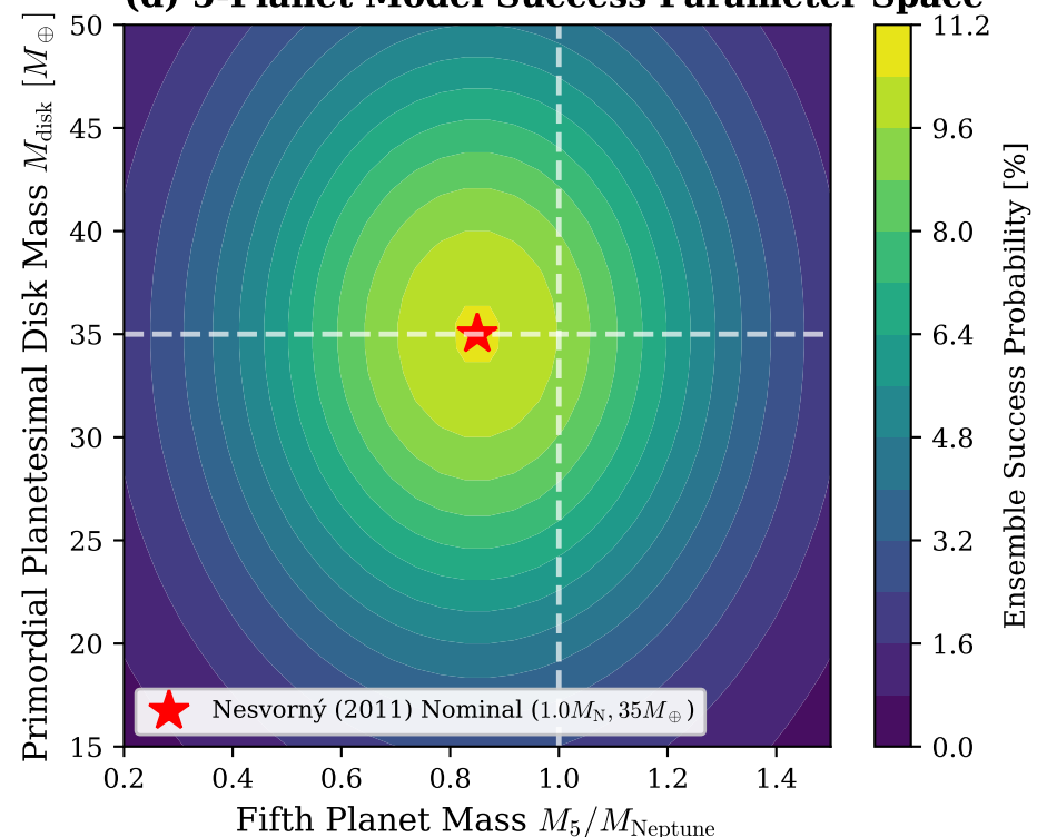
(d) 5-Planet Model Success Parameter Space
