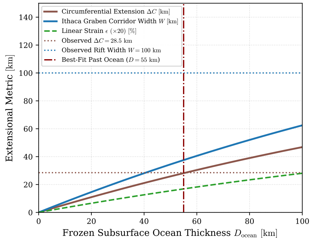
(d) Ocean Freezing & Ithaca Chasma Geometry
